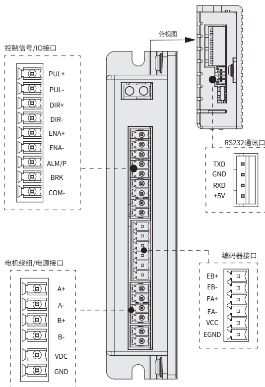
图 3-5 端子接口分布示意图
