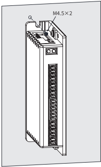
图 2-3 驱动器安装方式示意图
