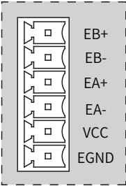
图 3-8 编码器信号接口示意图
