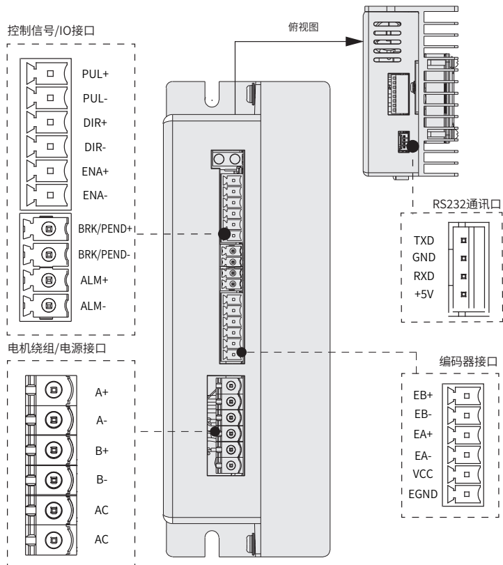
图 3-6 端子接口分布示意图
