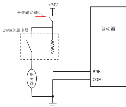
图 3-15 固态继电器接抱闸电机
