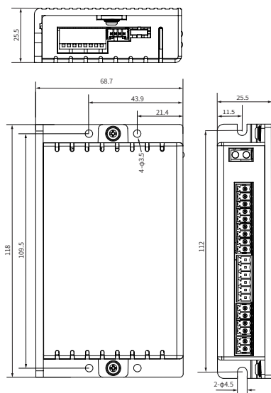
图 2-1 驱动器安装尺寸图 (单位: mm)
