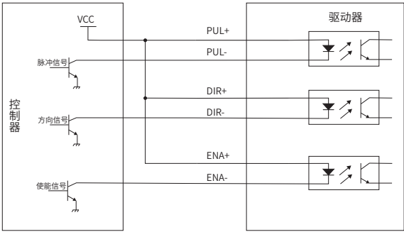
图 3-12 单端方式共阳极接法示意图
