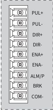
图 3-9 控制信号 /IO 端口示意图
