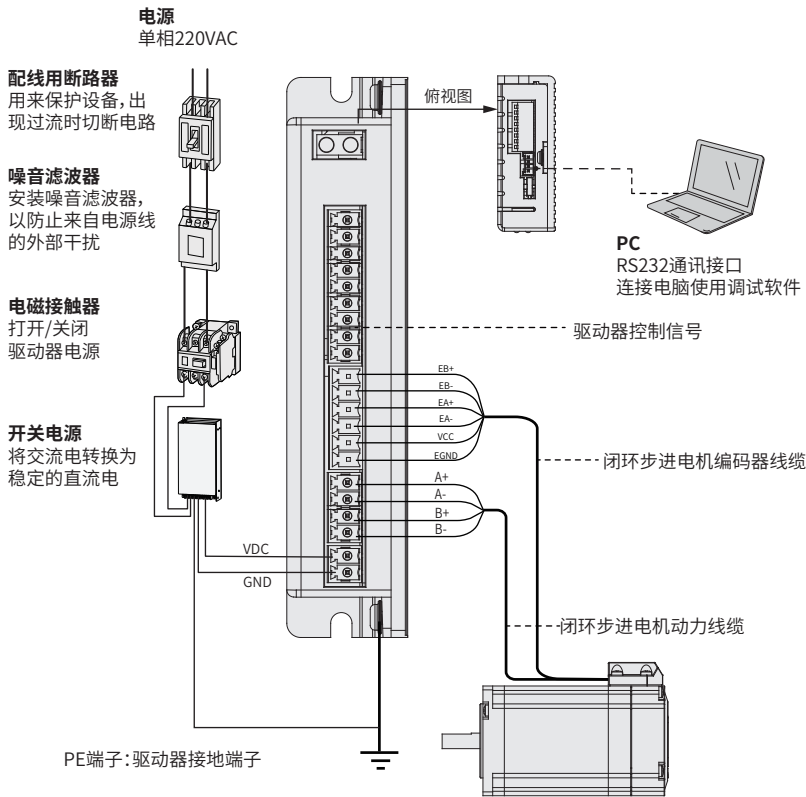
图 3-1 系统接线图
