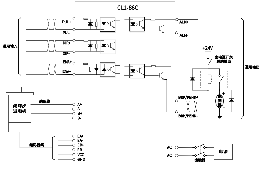
图 3-4 电气接线示意图
