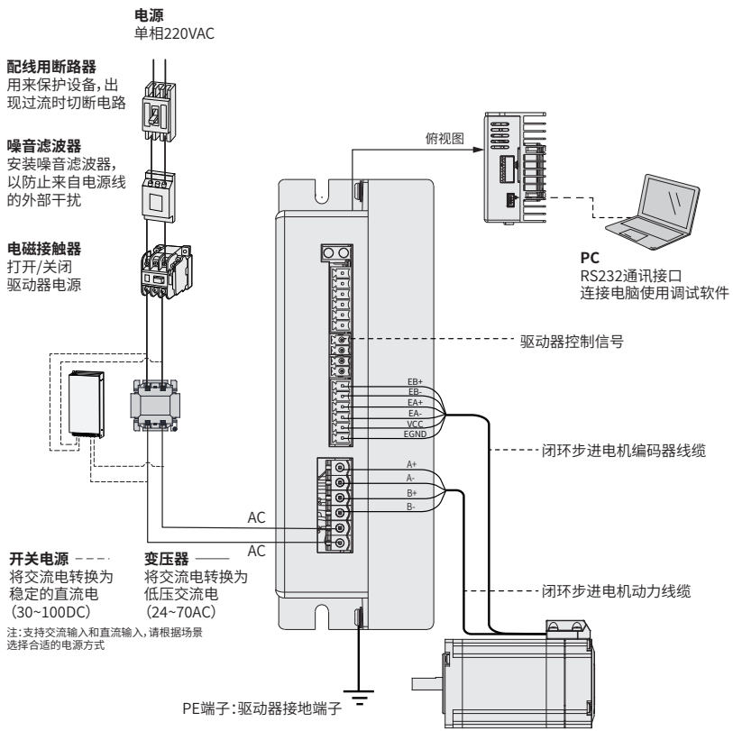
图 3-2 系统接线图
