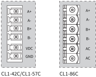
图 3-7 电机绕组和电源端子示意图
