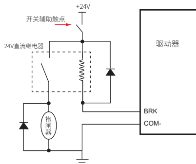
图 3-14 普通继电器接抱闸电机
