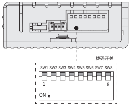
图 4-1 驱动器的拨码开关示意图
