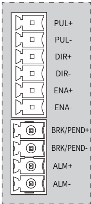
图 3-10 控制信号 /IO 端口示意图
