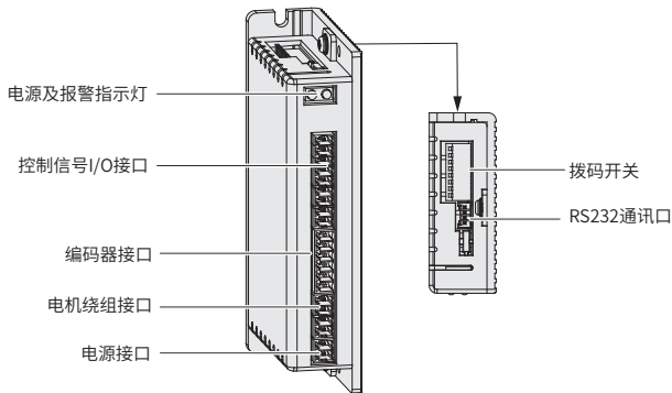
图 1-2 驱动器部件说明示意图
