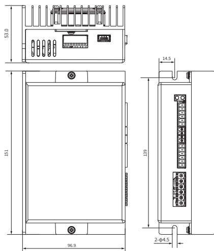
图 2-2 驱动器安装尺寸图 (单位: mm)
