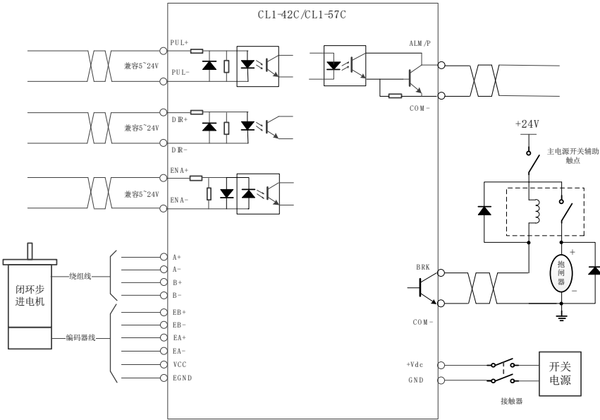
图 3-3 电气接线示意图
