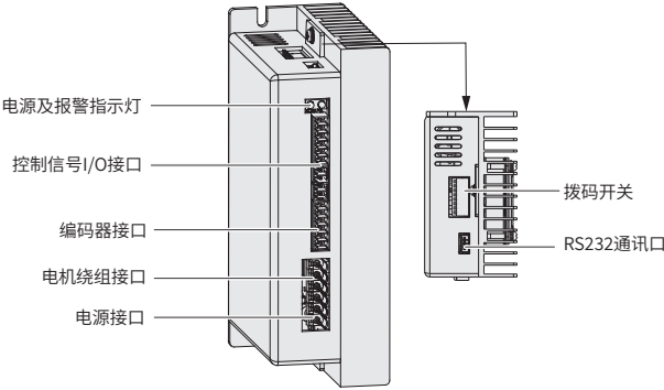
图 1-3 驱动器部件说明示意图
